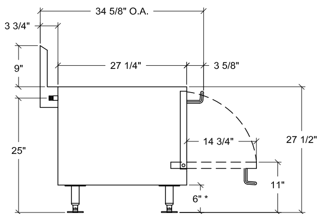
ÉLÉVATION FINALE
